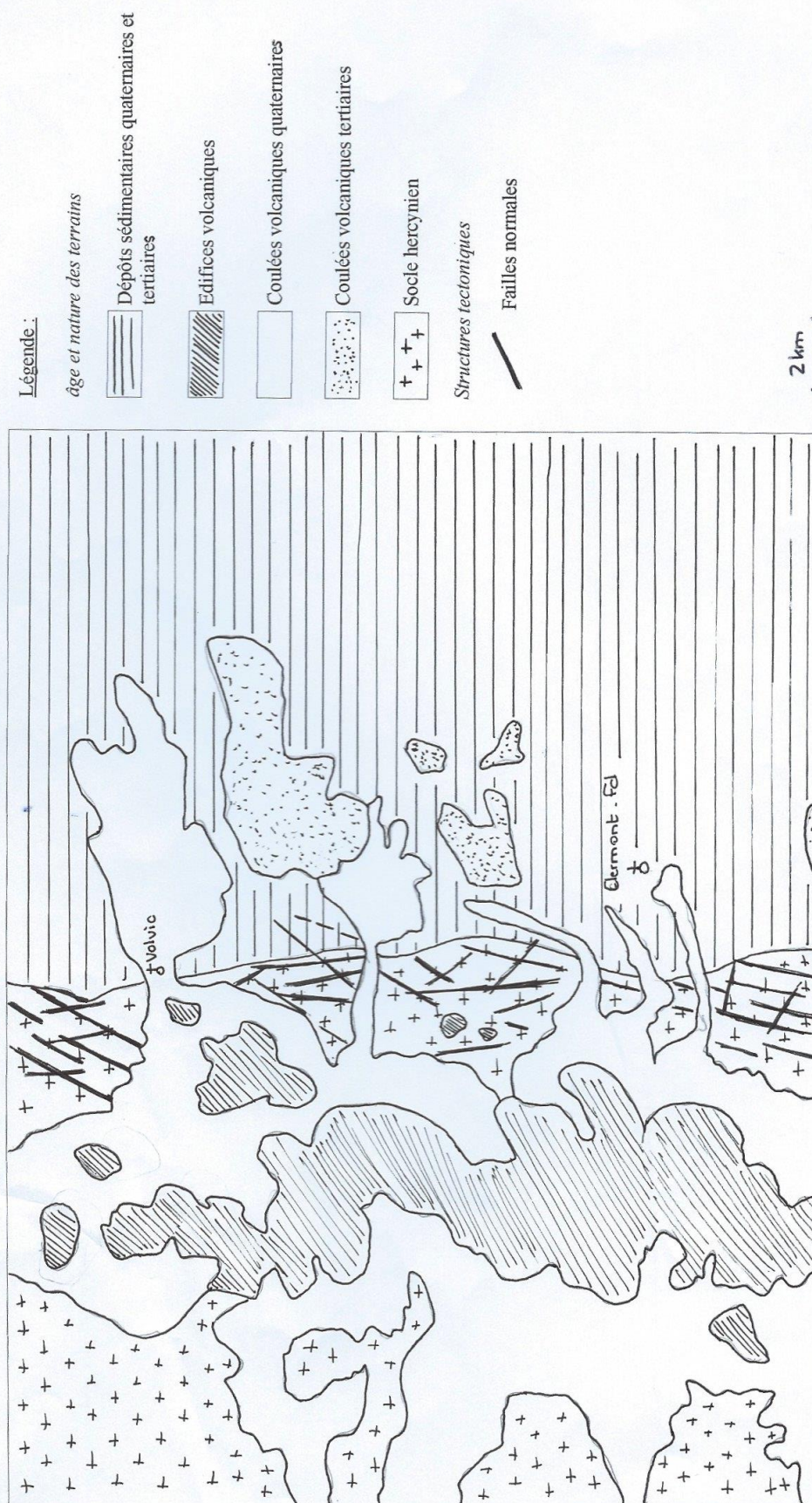
Schéma structural de la carte de CLERMONT-FERRAND (1/50 000e)
